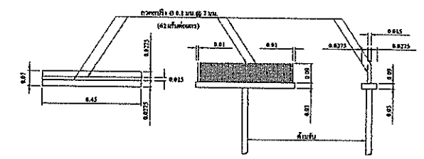
แบบขยายไม้ก่อคาลากผิวพื้น คสล. SCALE 1:25
