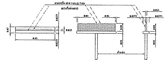
แบบขยายไม้กวางคอกผิวพื้น คสล. SCALE 1:25
