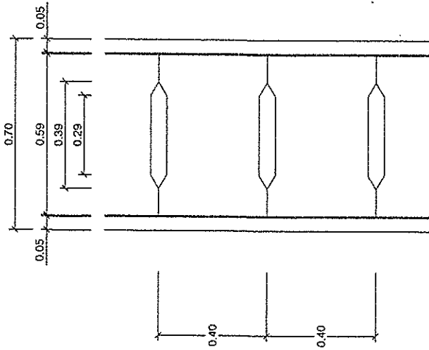
รูปแปลนวางระบายน้ำรูปตัวยูและฝาด
