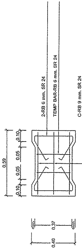
รูปขยายการเสริมเหล็กในฝาด
