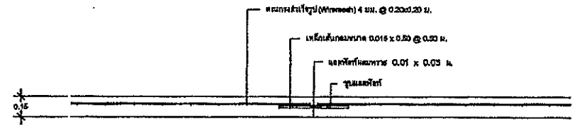
แบบขยาย contraction joint SCALE 1:25
