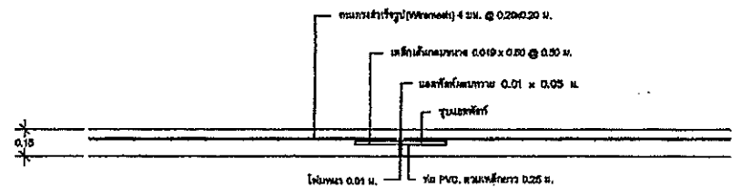
แบบขยาย expansion joint SCALE 1:25
