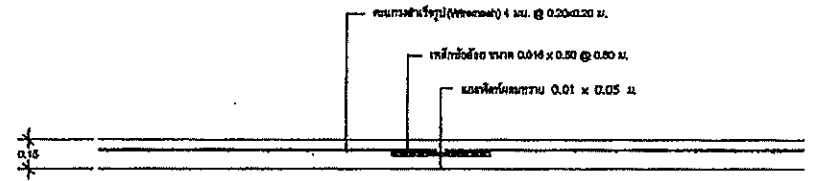
แบบขยาย longitudinal joint SCALE 1:25
