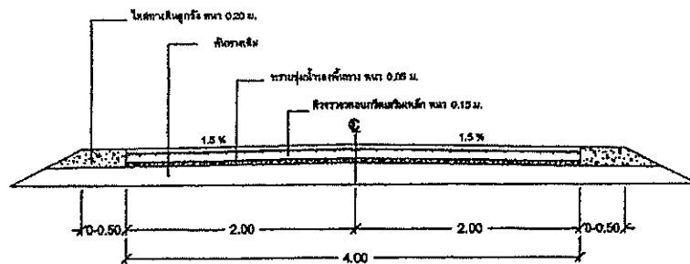
รูปตัด SCALE 1:50
