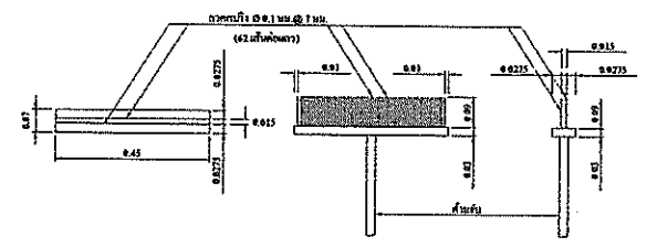
แบบขยายไม้กวดค้ำผิวพื้น คสล. SCALE 1:25
