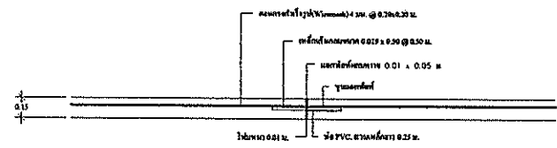
แบบขยาย expansion joint SCALE 1:50
