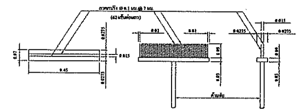
แบบขยายไม้กวางค้ำจายค้ำพื้น คสล. SCALE 1:25
