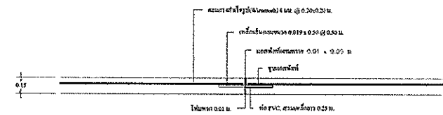
แบบขยาย expansion joint SCALE 1:50
