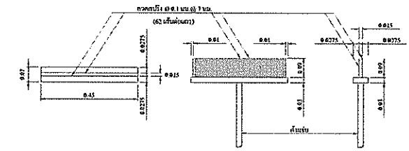
แบบขยายไม้กวดลากผิวพื้น คสล. SCALE 1:25
