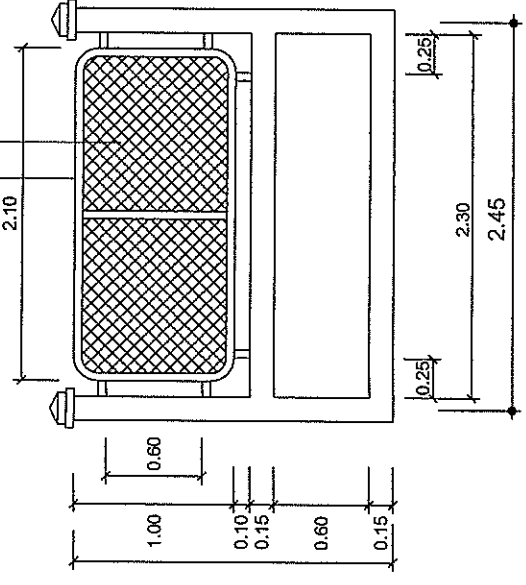
รูปด้านรั้วแบบที่ 1
